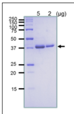
図. 精製した大腸菌 RuvB タンパク質の SDS-ポリアクリルアミドゲル電気泳動
